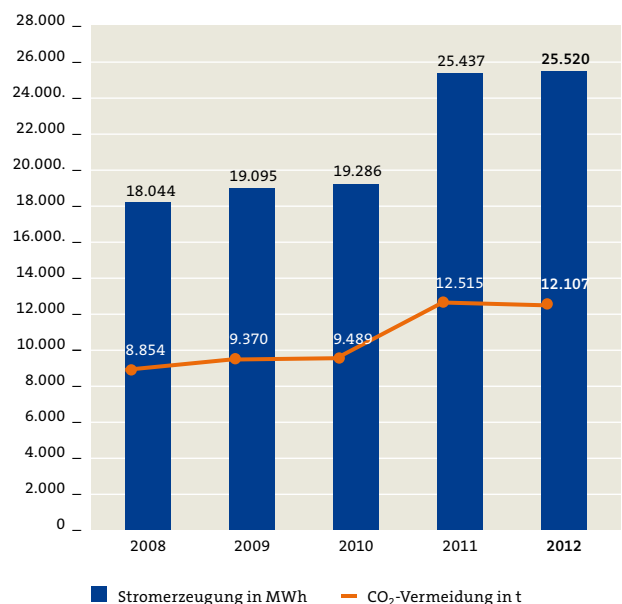
Stromerzeugung und CO 2 -Einsparung durch geförderte Fotovoltaikanlagen in eigenen und fremden Netzen
